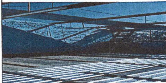
Foto 8: Desinstalación de lámina existente.
